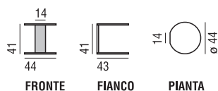
BLOG TAVOLINO ROTONDO design Lievore Altherr Molina (2006)
