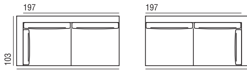
ANGOLO 220 SX A
