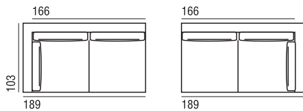
ANGOLO 189 SX A
